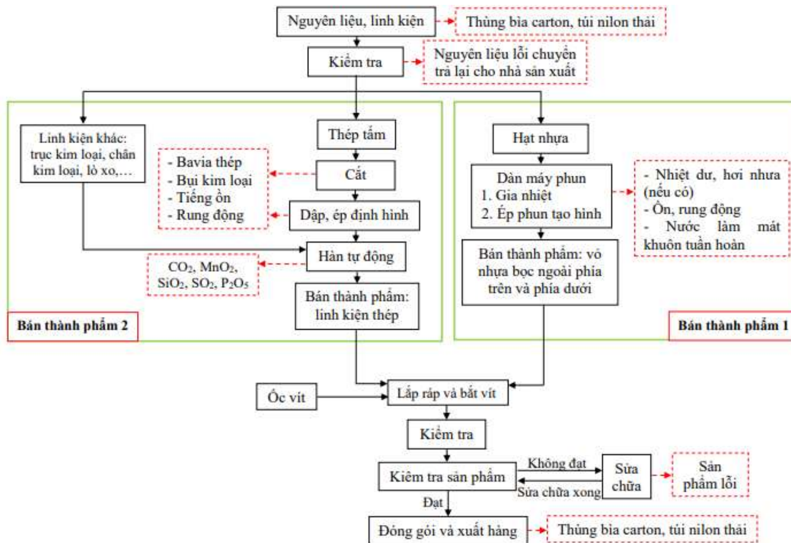
Hình 1.7. Quy trình sản xuất phần lõi của gói tựa đầu ô tô
