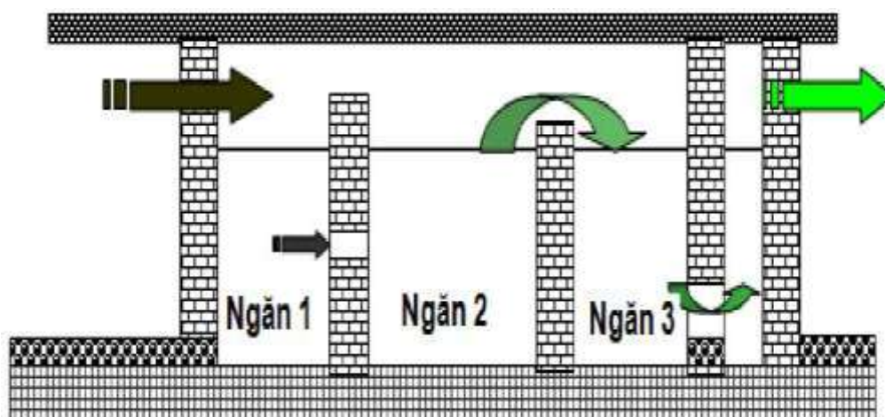
Hình 3.9. Sơ đồ cấu tạo của bể tự hoại 3 ngăn
