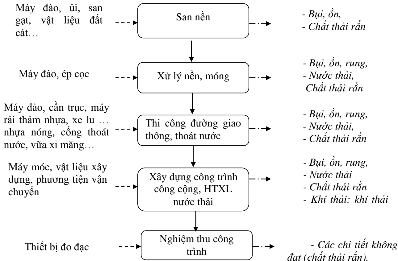
Hình 1. Quy trình thi công xây dựng
