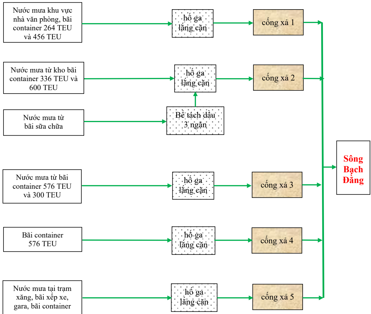
Hình 3.2. Sơ đồ các điểm thu gom, thoát nước mưa tại cơ sở
