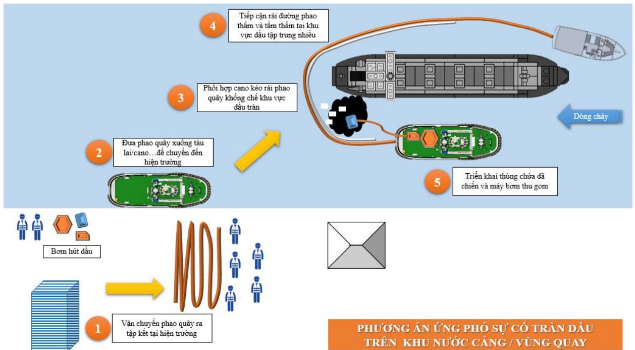
Hình 3.12. Quy trình ứng phó SCTD khu nước trước cầu cảng
