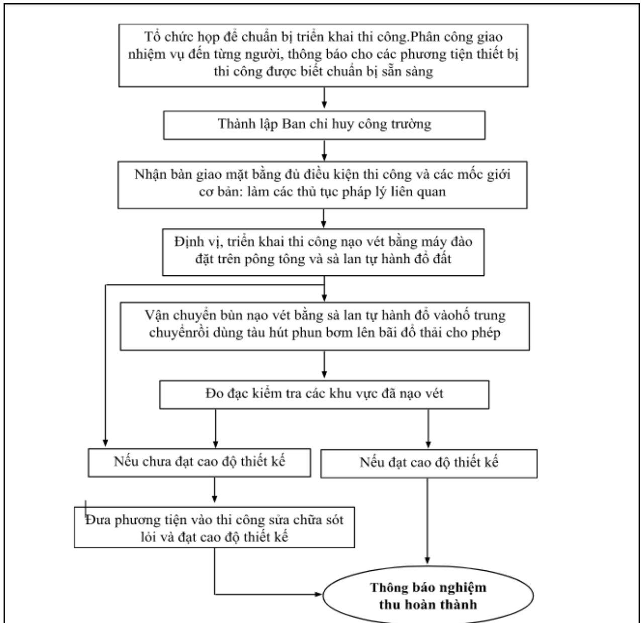
Hình 1.12. Sơ đồ phương án thi công nạo vét định kỳ
