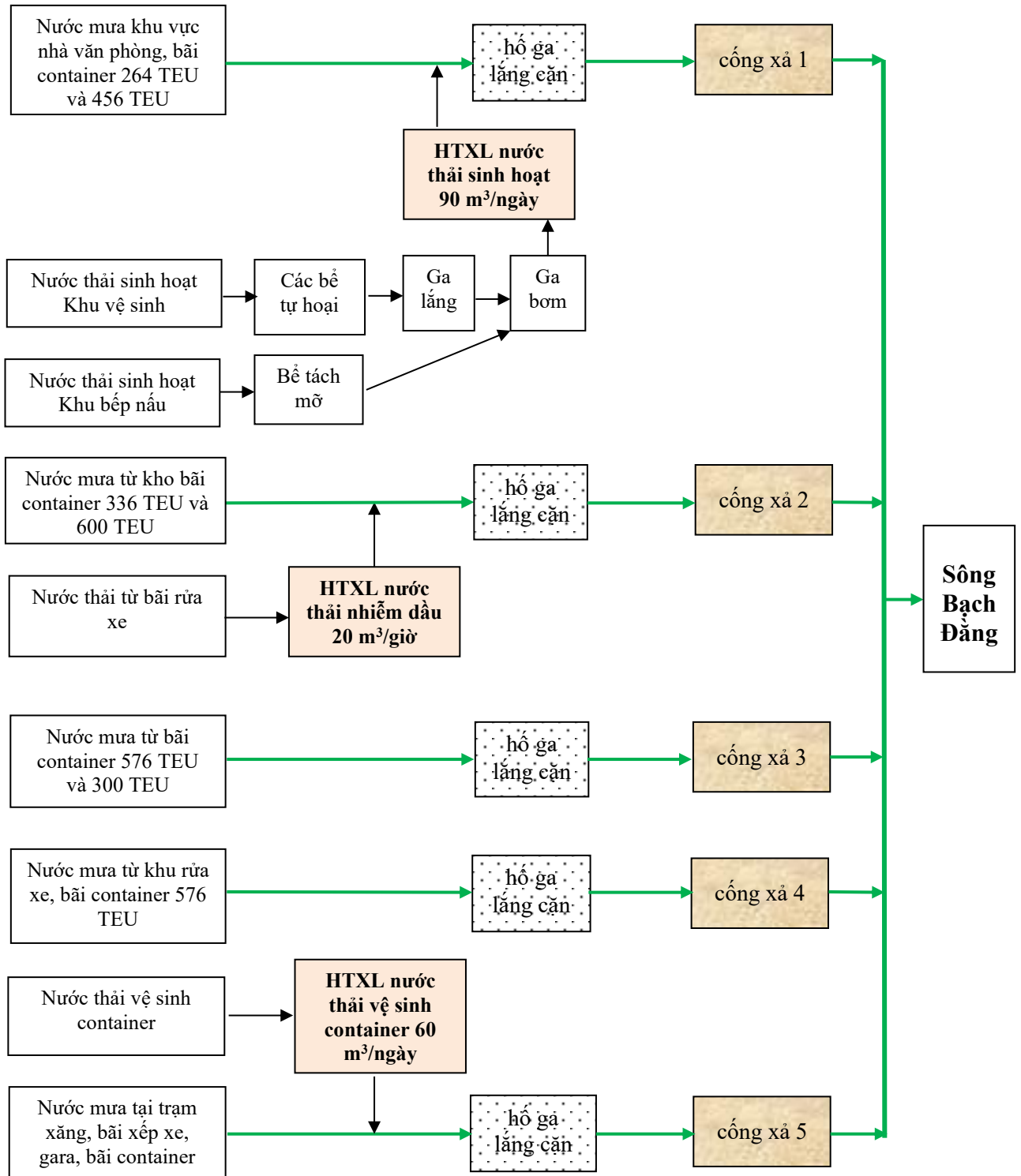
Hình 3.3. Sơ đồ thu gom, thoát nước thải tại cơ sở
