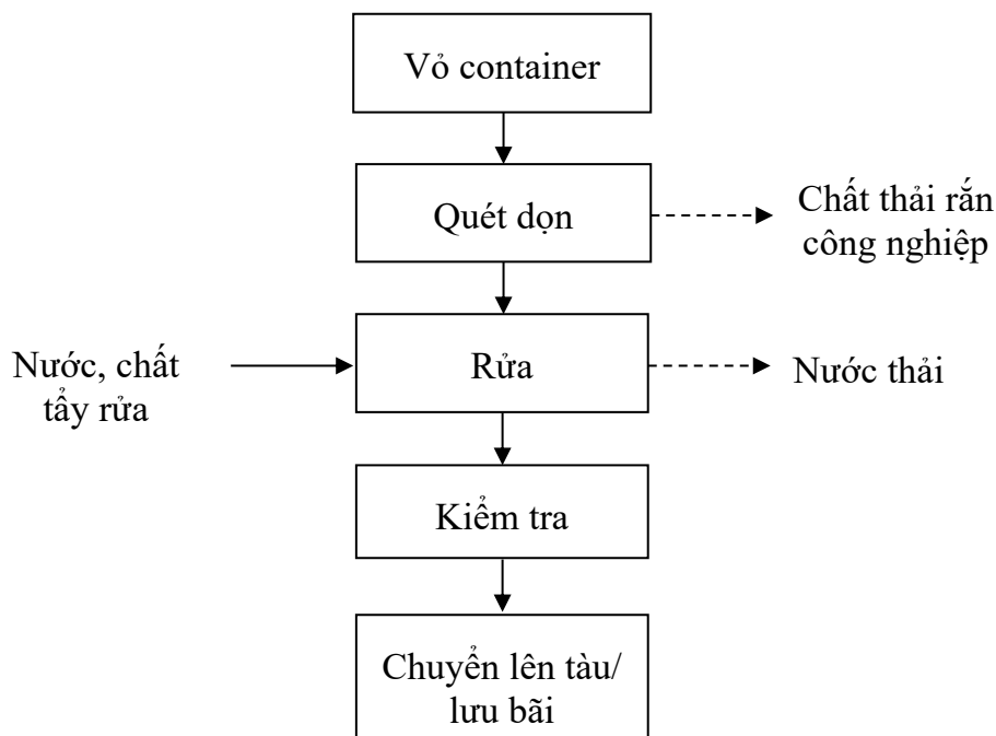
Hình 1.11 Sơ đồ các bước vệ sinh vỏ container
