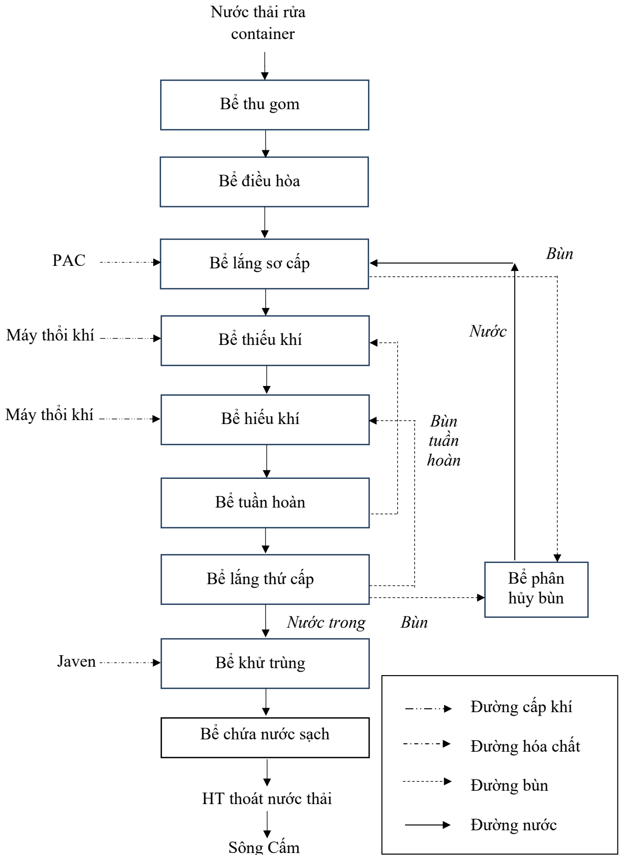
Hình 3.8. Quy trình công nghệ HT xử lý nước thải rửa container
